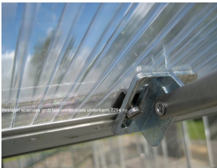
2295: Beslaget spændes godt fast om vinduets underkarm (Zeus 7293, Helena 7366).
